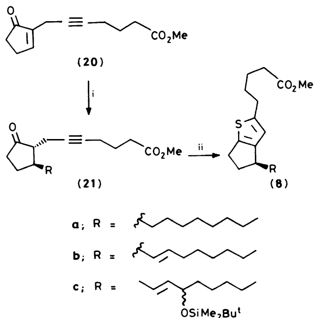
Scheme 3. Reagents: i , 'RCu'; ii , \text{H}_2\text{S}
